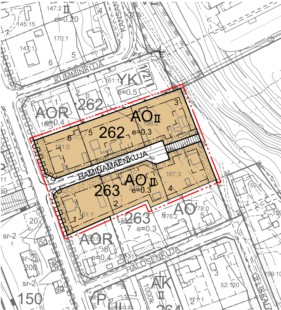
Asemakaavaluonnos 1:2000
